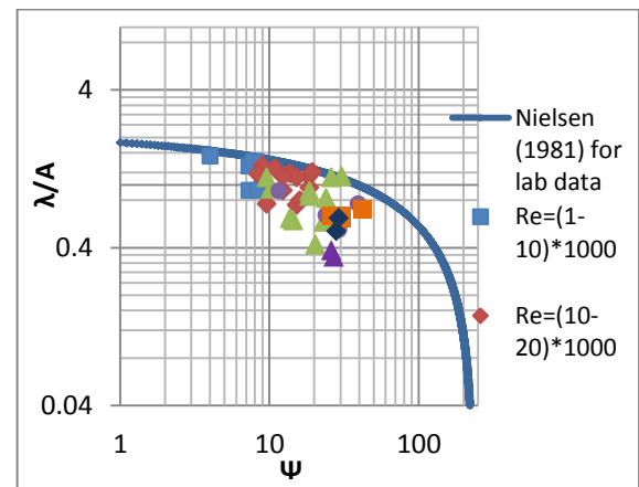
شکل (۷) مقایسه داده‌های آزمایشگاهی طول موج بدون بعد ریپل برحسب اعداد رینولدز مختلف با منحنی نیلسن (۱۹۸۱) برای داده‌های آزمایشگاهی.
