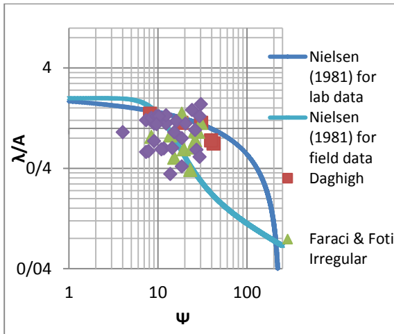
شکل (۶) طول موج بدون بعد ریپل اندازه گیری شده روی منحنی‌های نیلسن (۱۹۸۱) برای داده‌های آزمایشگاهی و میدانی.
