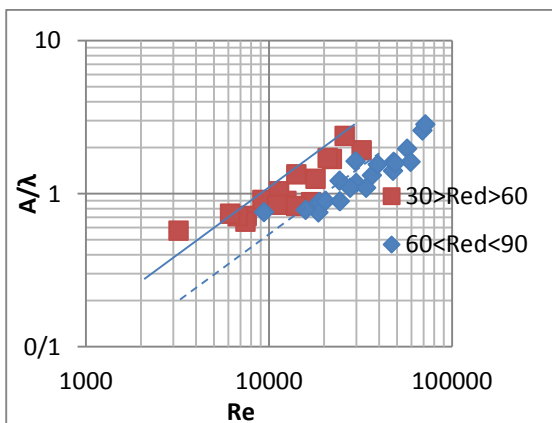
شکل (۸) رابطه دو پارامتری پیشنهادی برای طول موج بدون بعد ریپل.
