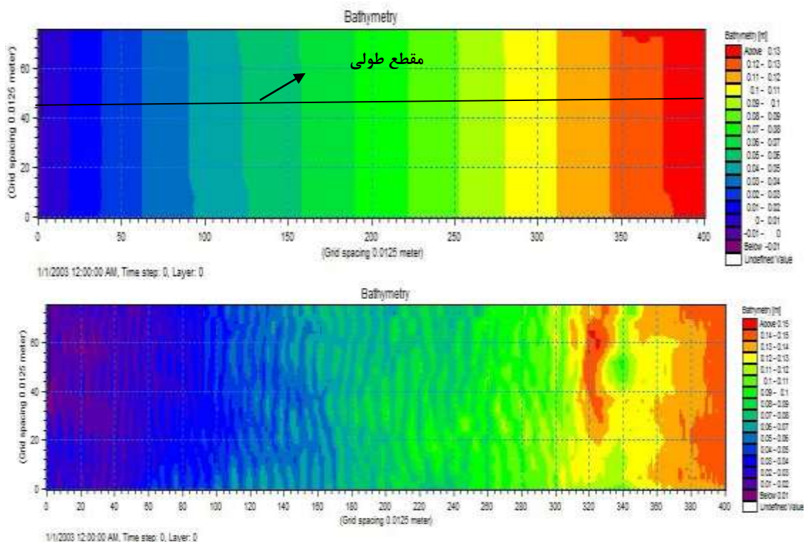
شکل (۴) الف) پروفیل بستر قبل از موج و ب) پروفیل بستر بعد از موج با ارتفاع ۰/۱۱ متر و پریود ۲/۲ ثانیه.
