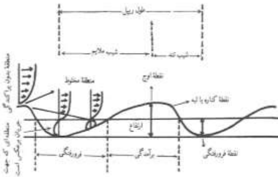
شکل (۱) شکل هندسی ریپل مارک‌ها همراه با پراکندگی انرژی (سرعت) در رابطه با حرکت ذرات معلق در روی آن‌ها.
