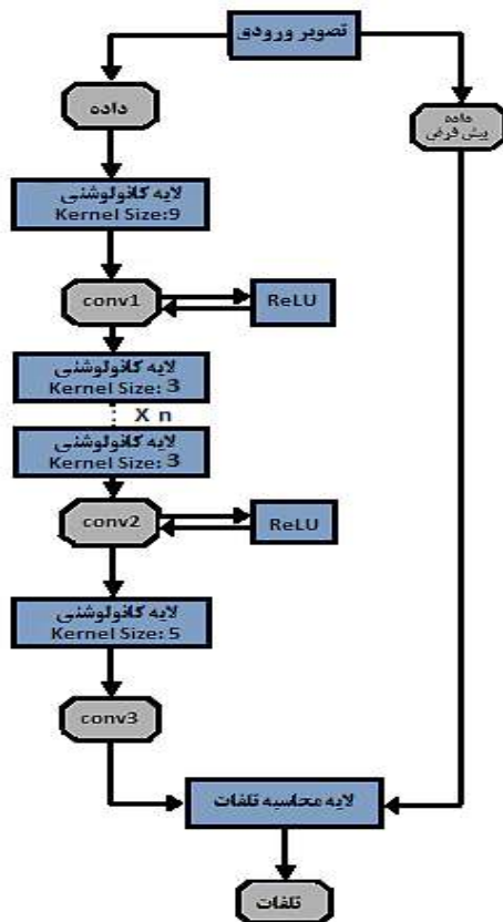
شکل (۵) بلوک دیاگرام شبکه عصبی CNN.
