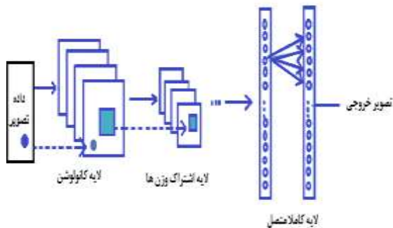
شکل (۲) لایه‌های شبکه عصبی CNN.
