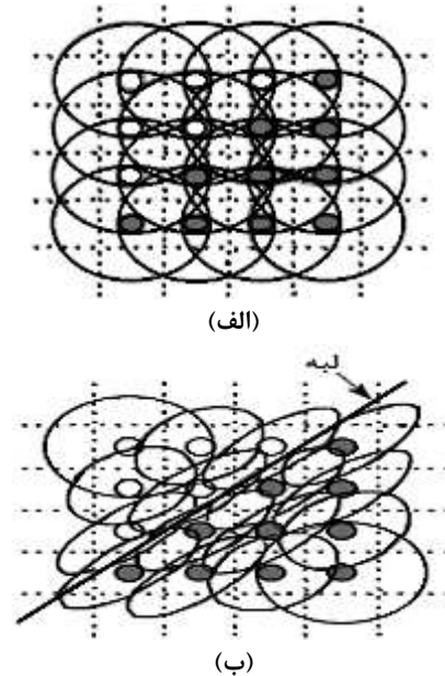
شکل (۶) (الف) کرنل‌های استاندارد و (ب) کرنل‌های استرینگ در امتداد لبه [۹].
