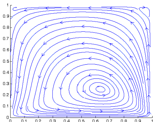
شکل (۹) مسیر تقریبی جریان برای مثال ۲ به ازای Re=100 در زمان t=1 که با استفاده از توابع شعاعی بدست آمده است.
