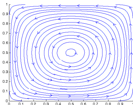
شکل (۳) مسیر دقیق خطوط جریان برای مثال ۱ به ازای Re=100 در زمان t=1 .
